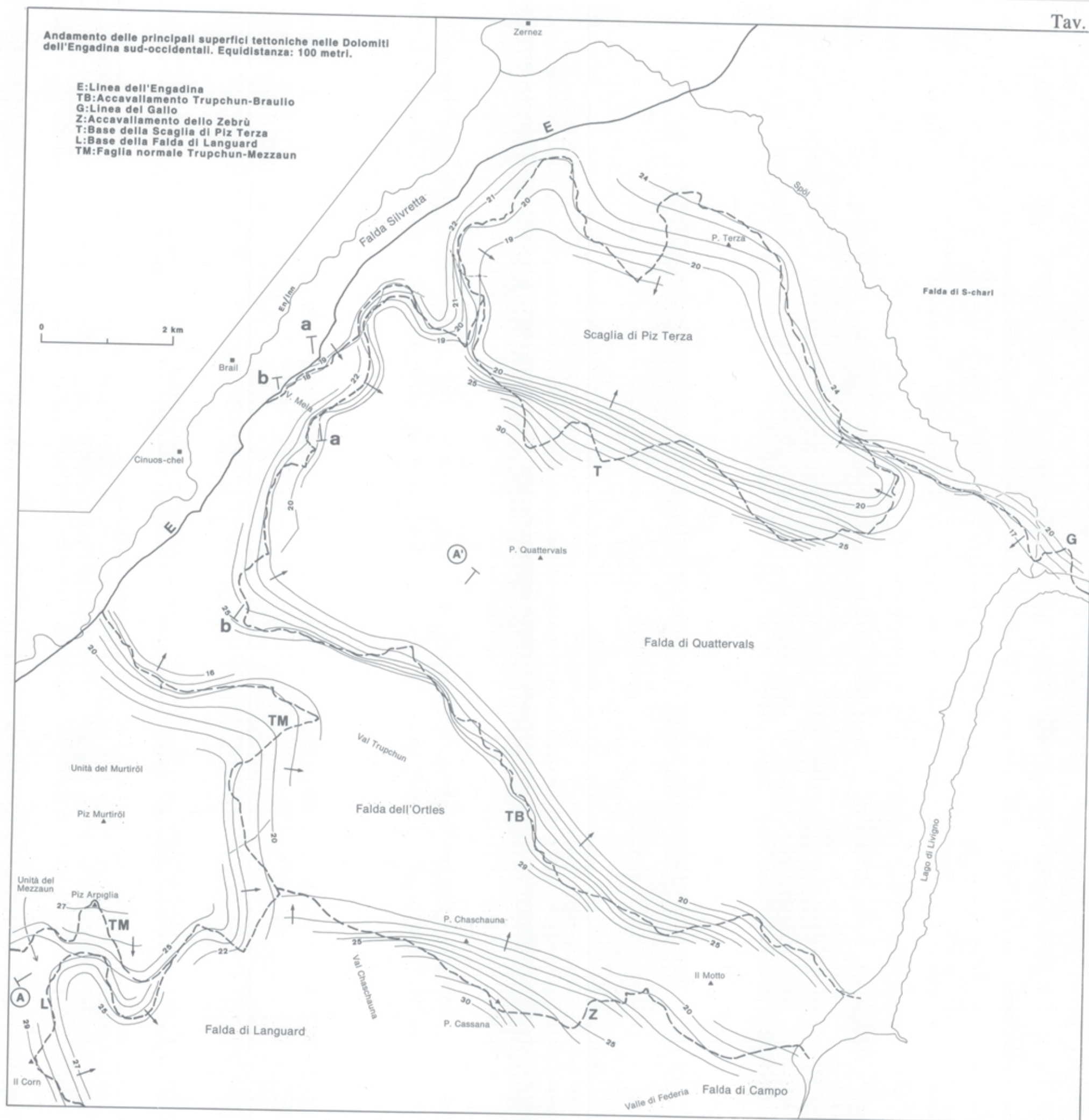
Tav. 2 - Andamento delle principali superfici di accavallamento nella parte SW delle Dolomiti dell'Engadina.
