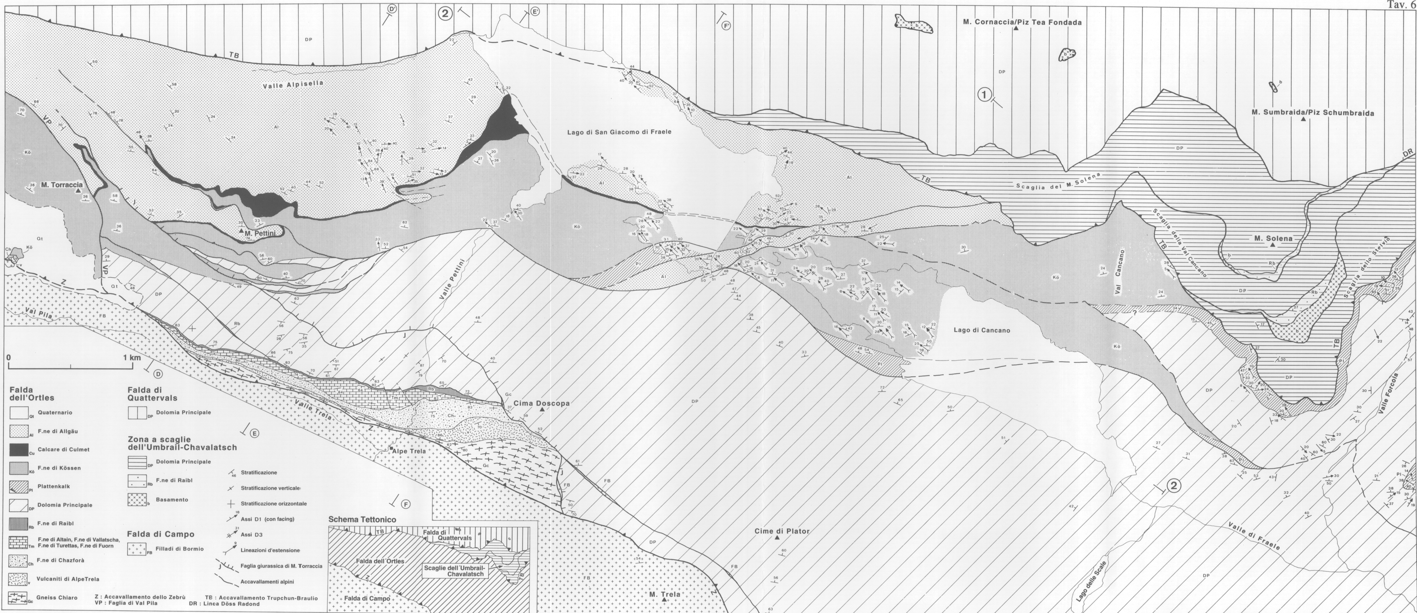
Tav. 6 - Carta geologico-strutturale dell'area M. Torraccia-Valle Forcola. Rilevamento P. CONTI, G. MANATSCHAL. - Geological map of the M. Torraccia-Valle Forcola area. (P. CONTI & G. MANATSCHAL).
