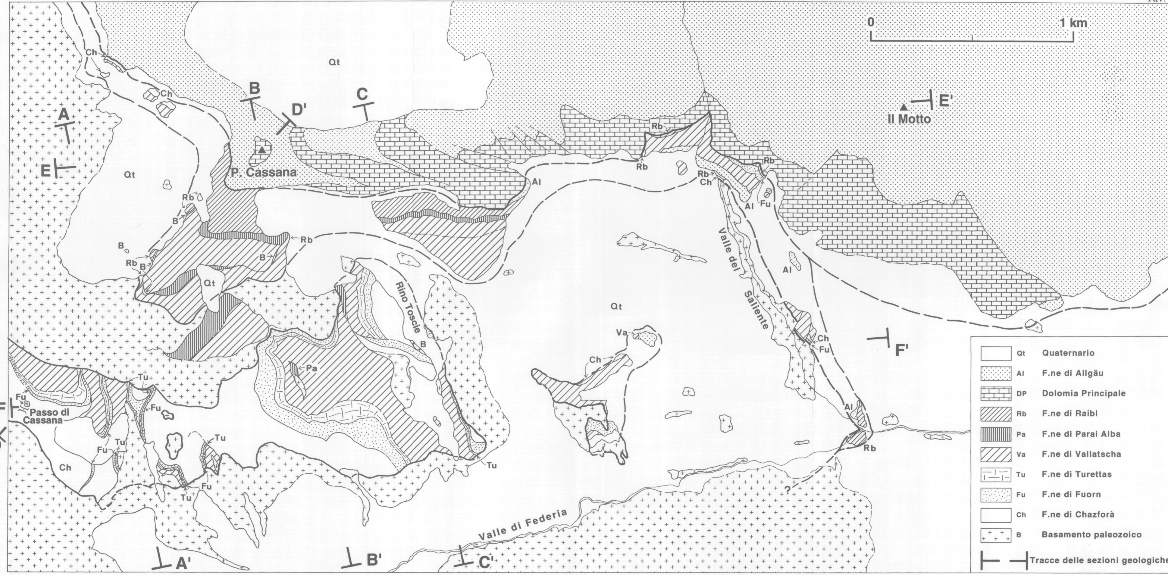
Tav. 9 - Carta geologica dell'area P. Cassana-II Motto. - Geological map of the P. Cassana-II Motto area.
