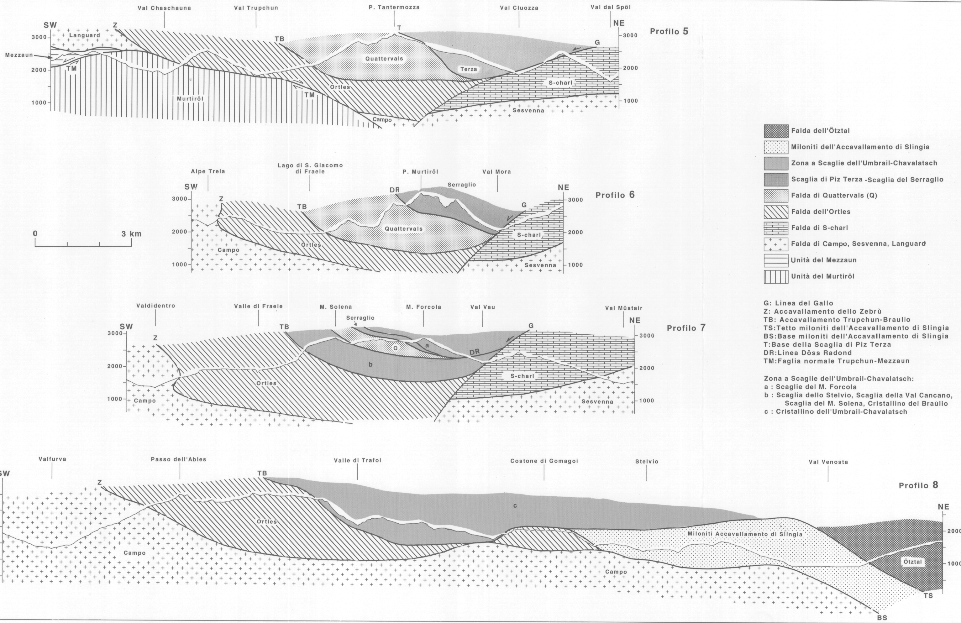
Tav. 14 - Profili attraverso le Dolomiti dell'Engadina. Per le tracce dei profili vedi fig. 33. - Profiles in the Engadine Dolomites area. See Fig. 33 for profile traces.
